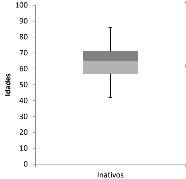
BOXPLOT INATIVOS
